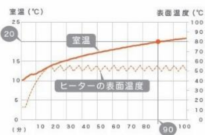
洗面室とヒーターの温度上昇データ
